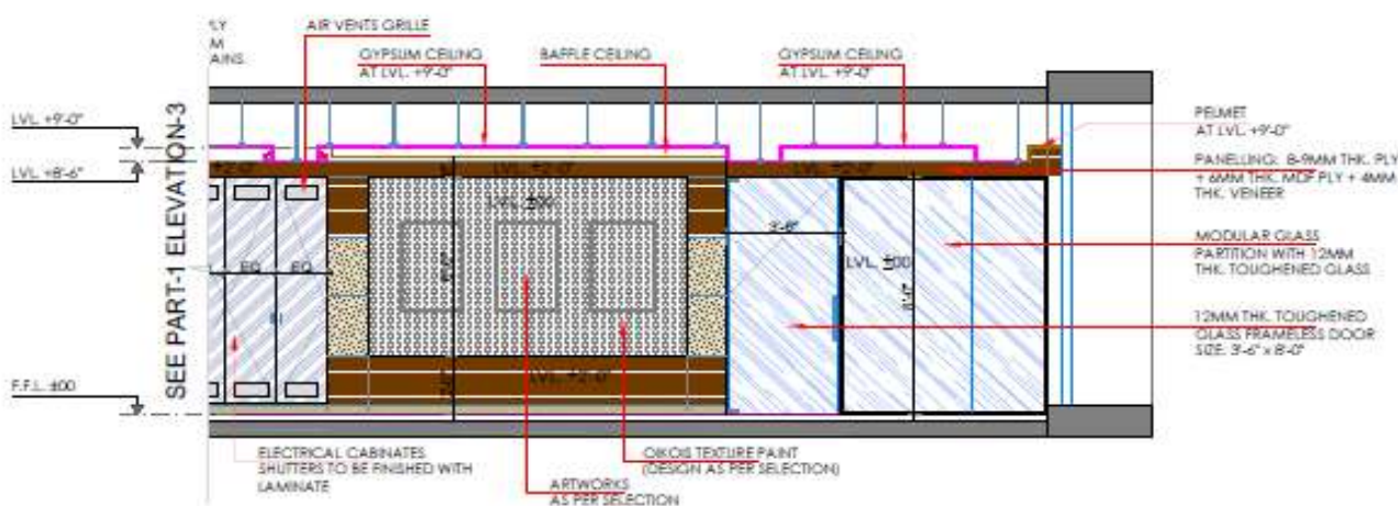
ELEVATION -3 (PART-2) (WAITING AREA & LOBBY)
